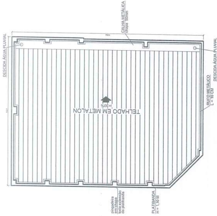
PLANTA DE COBERTURA ESC. 1 : 100
